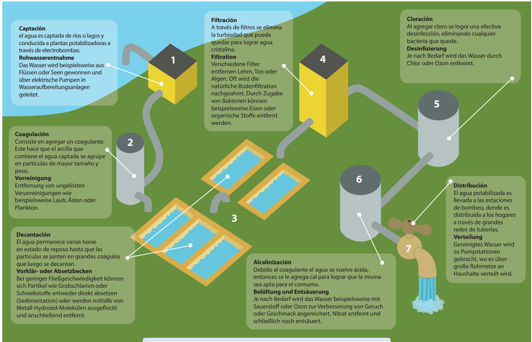
Sistema de tratamiento de agua potable en Costa Rica (Trinkwasseraufbereitung in Costa Rica)
